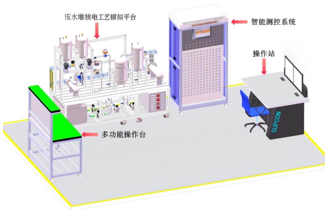
图 5-3 职工组（核电）竞赛工位布局图（参考）
